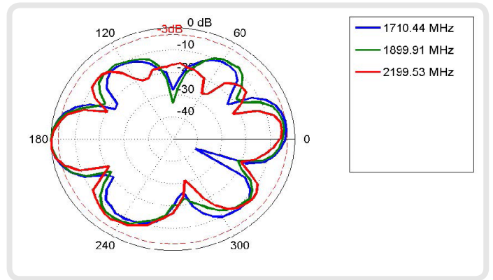
H-Plane: 1700 - 2200 MHz
